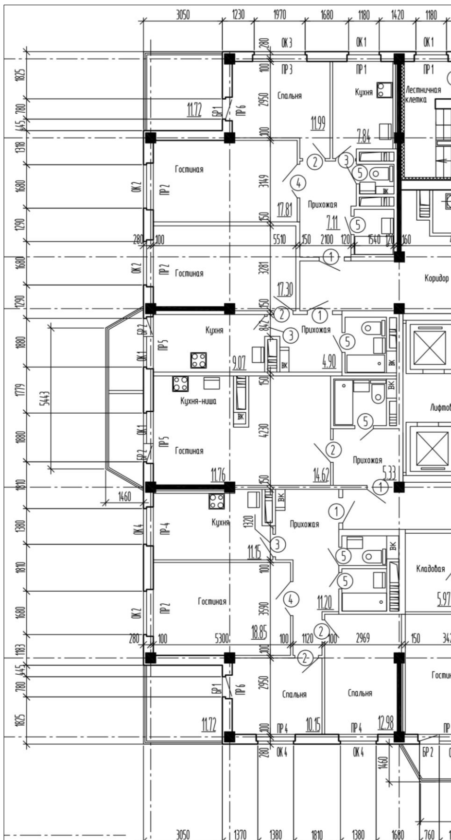
Рисунок 2 Фрагмент плана типового этажа
